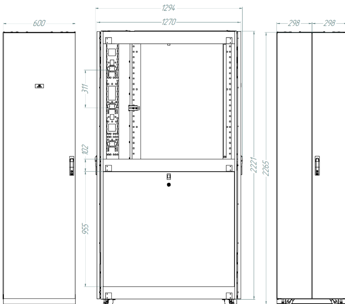
Вид спереди
