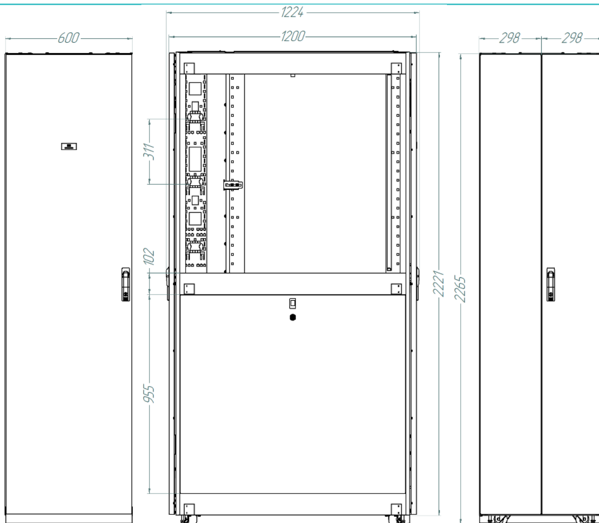
Вид спереди
