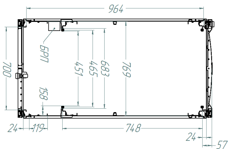
Сечение горизонтальное
