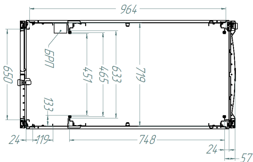
Сечение горизонтальное
