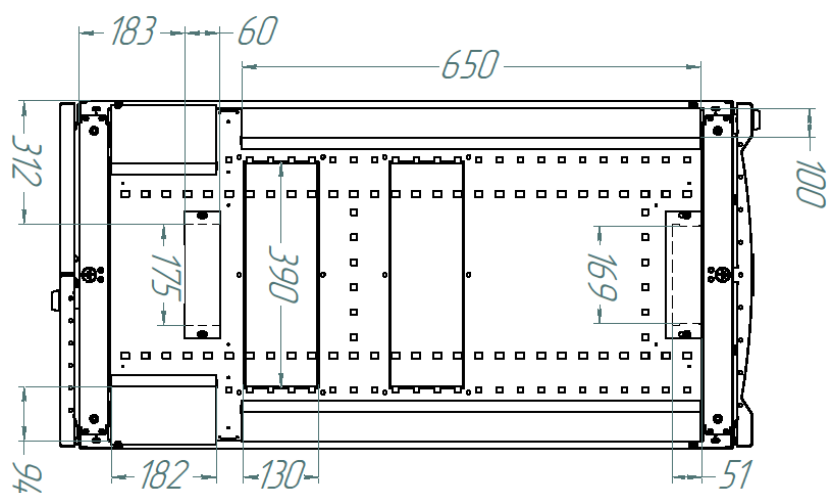
Вид сверху
